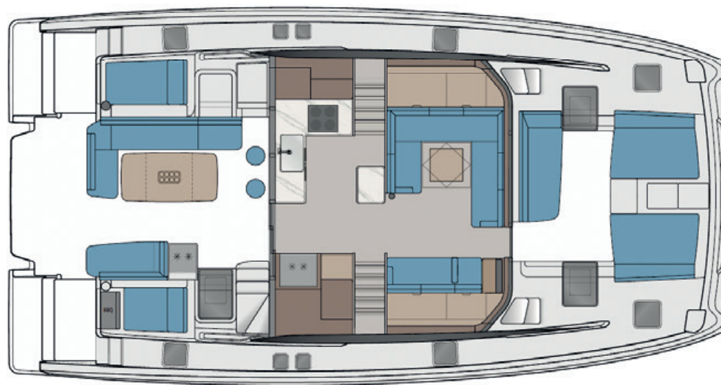
Standard-Hauptdeck SOFA STEUERBORD OPTIONAL
