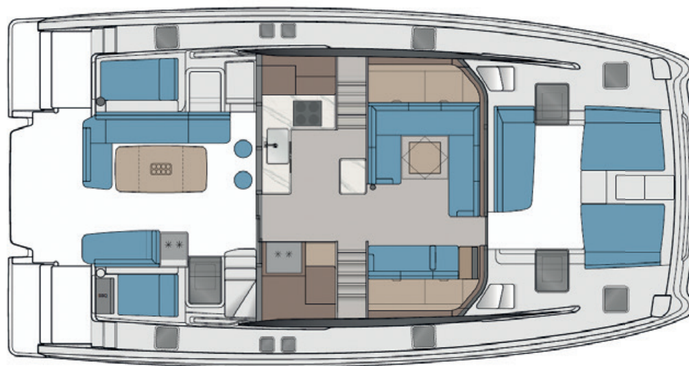
Standard-Hauptdeck Sofa Steuerbord optional
